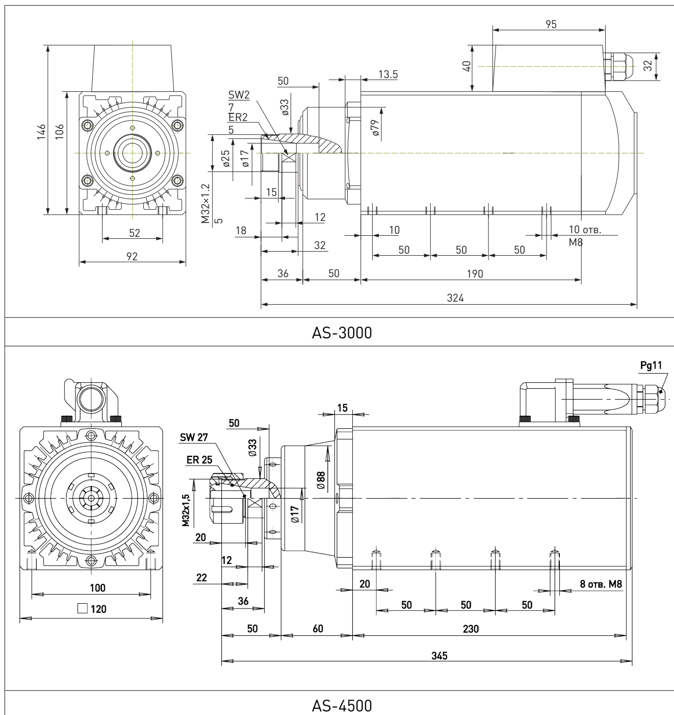
Рис. 2. Габаритные и установочные размеры шпинделей
