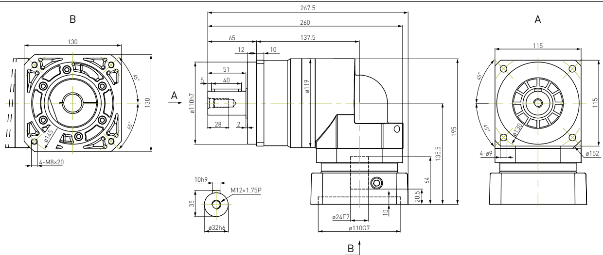
115EVB5K-S32-P0, 115EVB10K-S32-P0
