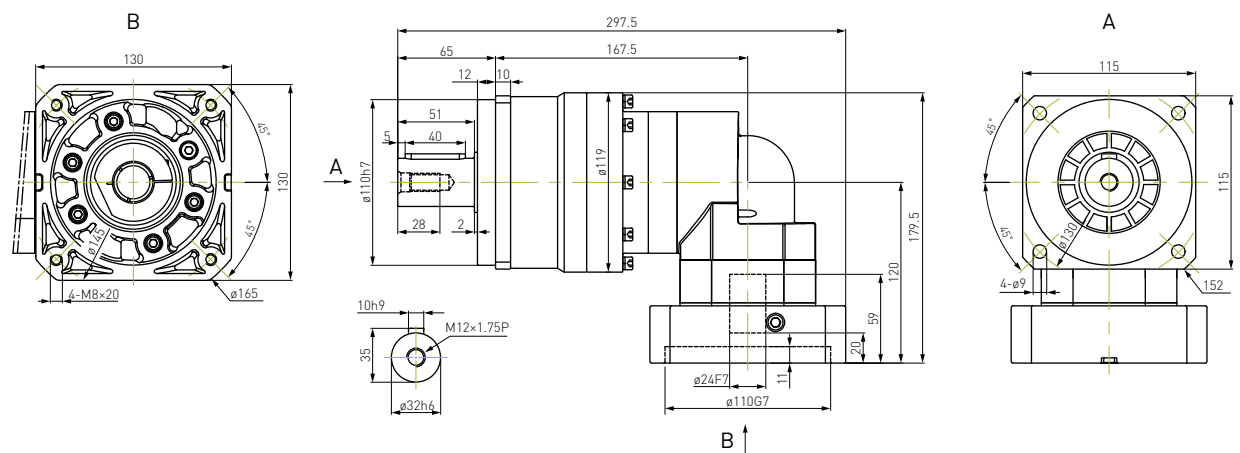
115EVB20K-S32-P0
