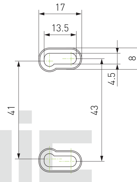
Монтажные отверстия (увеличенный вид)
