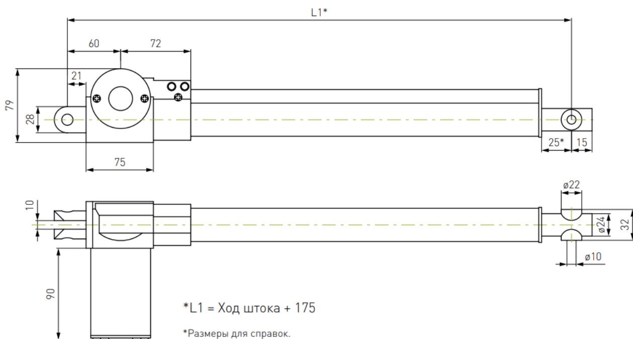
Рисунок 1 – Габаритные и присоединительные размеры (мм) актуаторов TGB.
