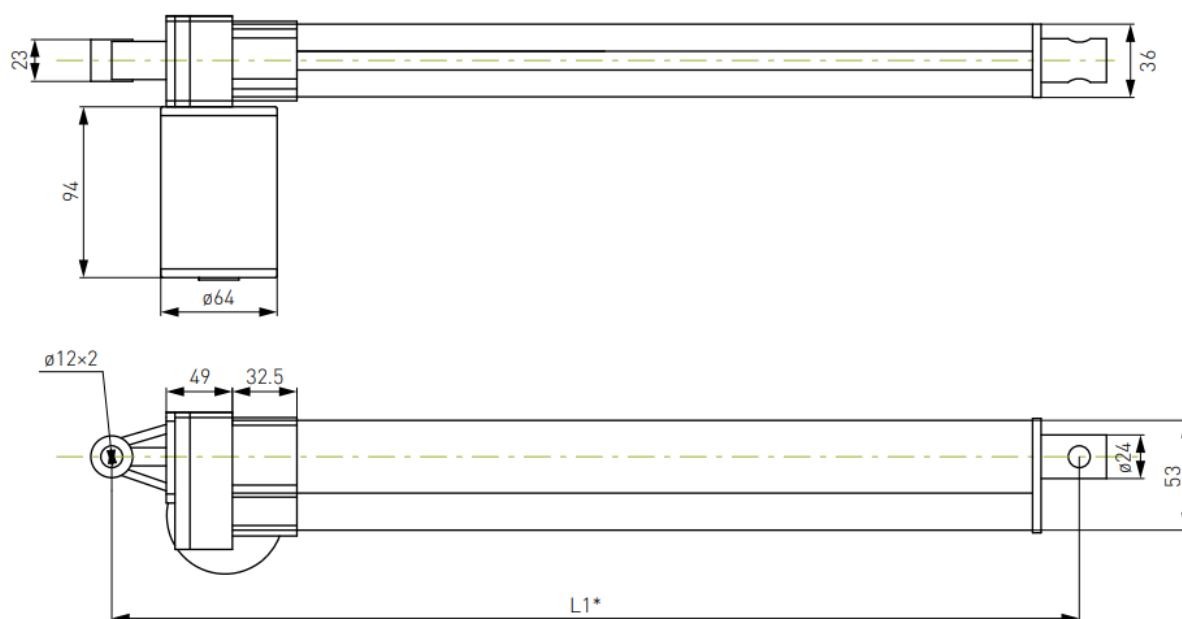
Рисунок 2 – Габаритные и присоединительные размеры (мм) актуаторов TGB-L.
