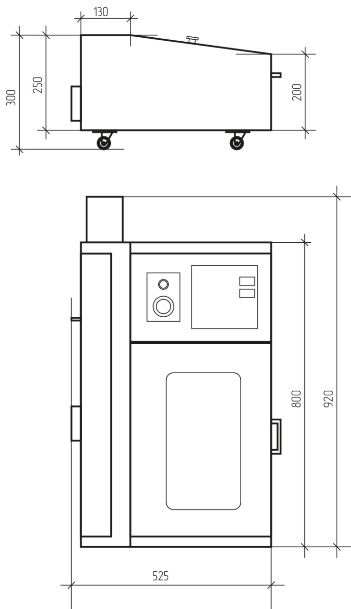
Рис. 1. Габаритные размеры LP320-50W
