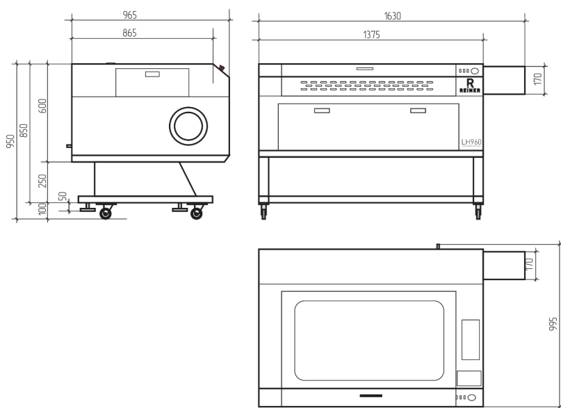
Рис. 1. Габаритные размеры LH960-100W/LP960-100W
